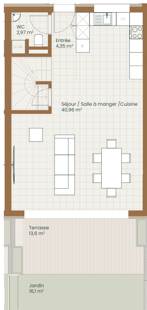
REZ-DE-CHAUSSÉE
